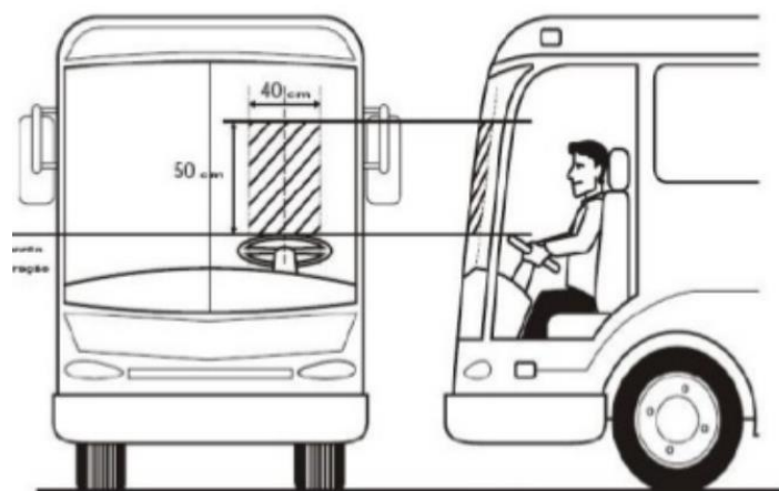
FIGURA 1: ILUSTRAÇÃO - ÁREA CRÍTICA DE VISÃO DO CONDUTOR
